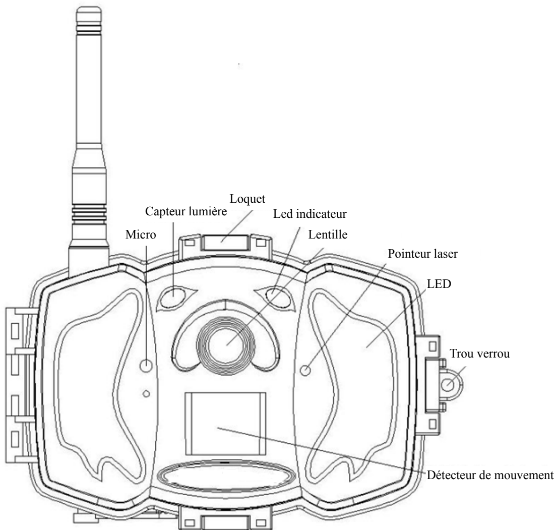
Figure 1 Diagramme des éléments de la caméra
