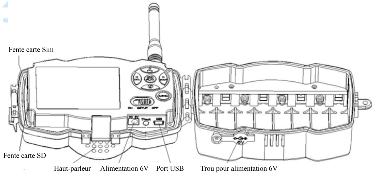
Figure 3 Diagramme de l'interface
