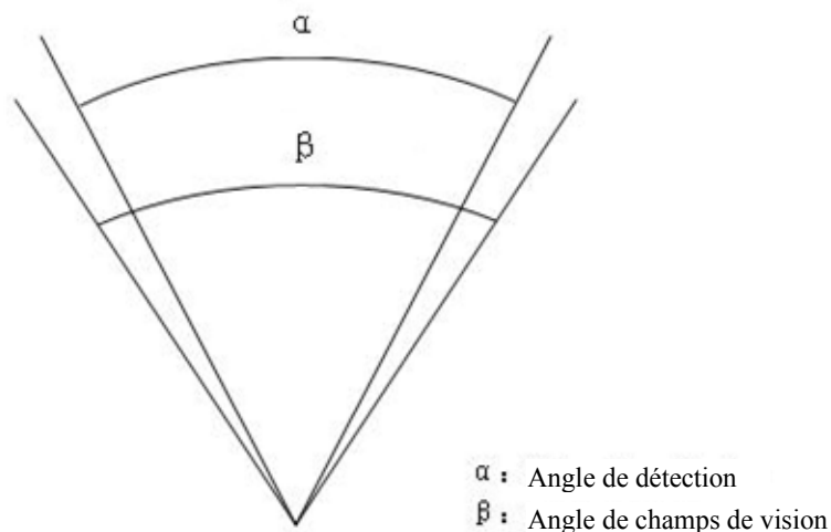
Figure 6 Angle de détection vs angle de champs de vision
