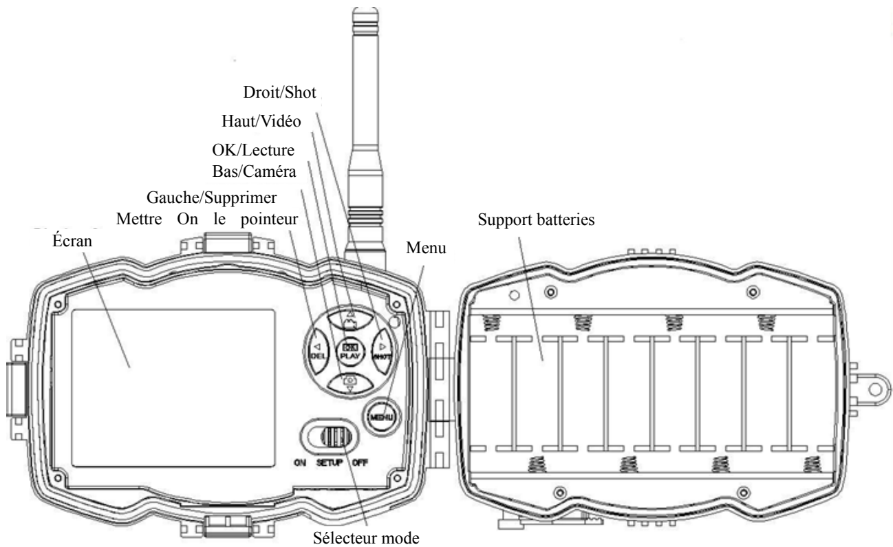
Figure 2 Intérieur de la caméra
