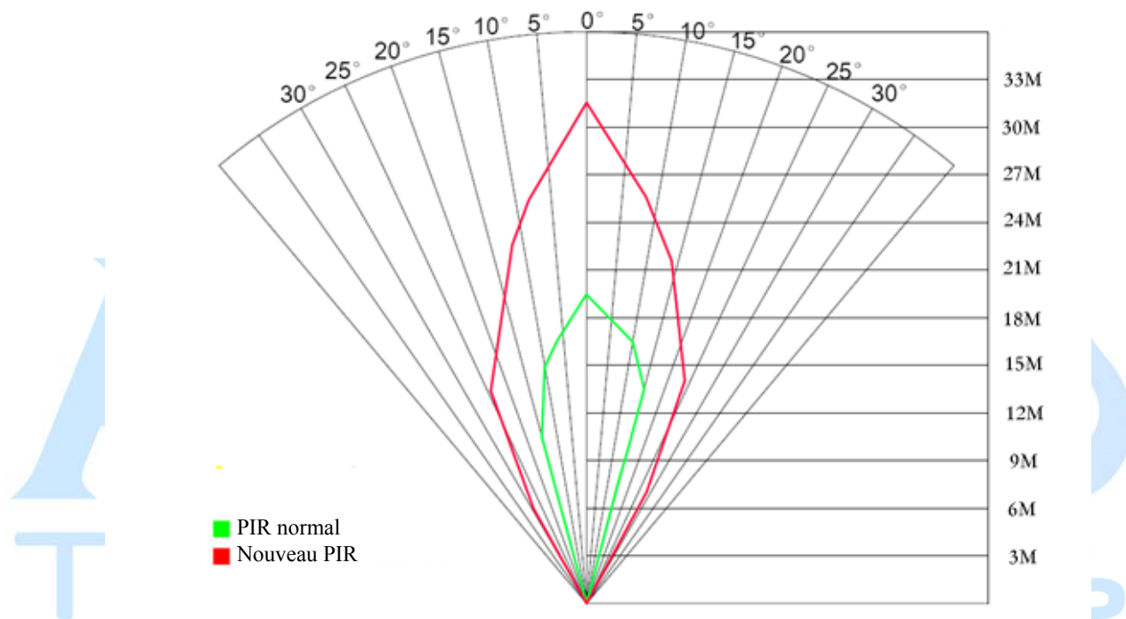
Figure 7 Comparaison des zones de détection du nouveau et existant PIR
